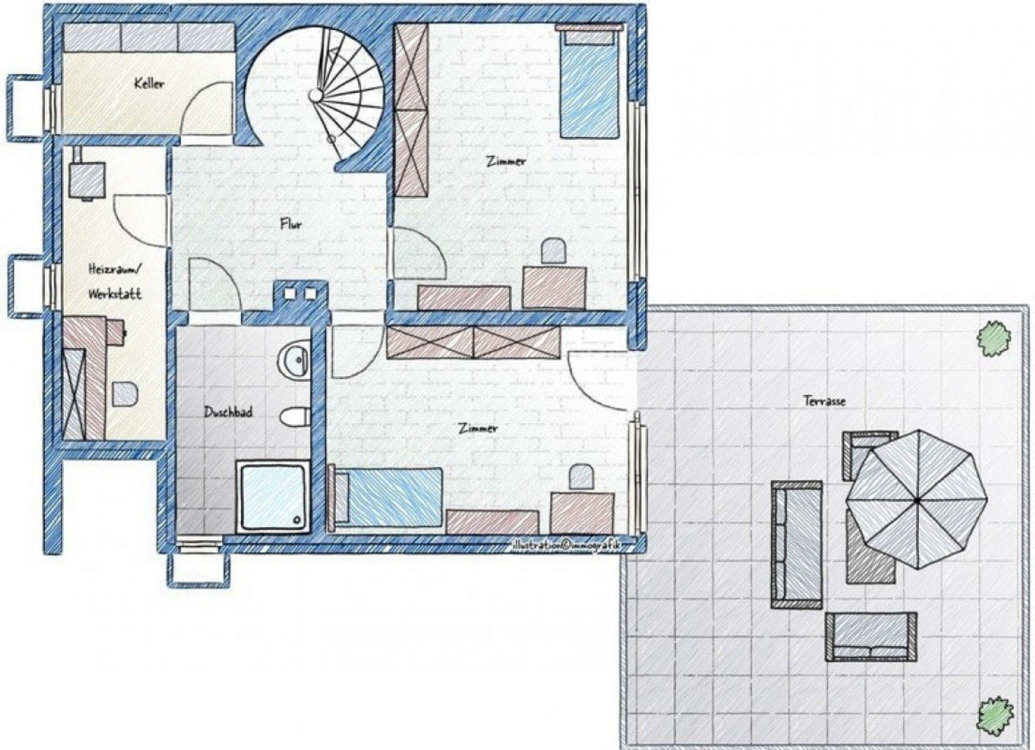
Grundriss Untergeschoss
