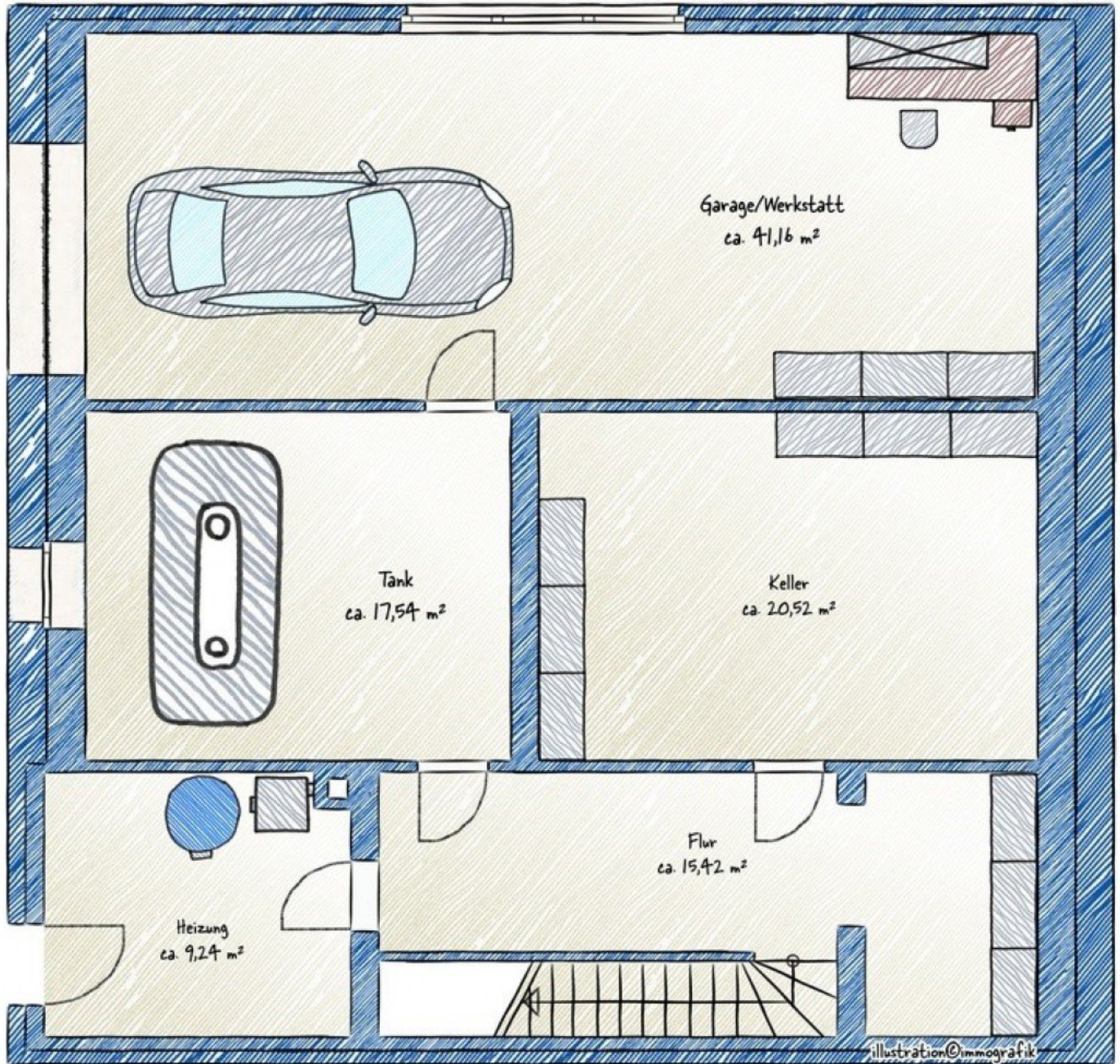
Grundriss Untergeschoss
